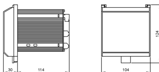
DIMENSIONI VERSIONE IP54
